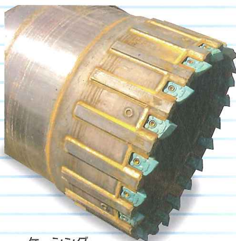
ケーシング
